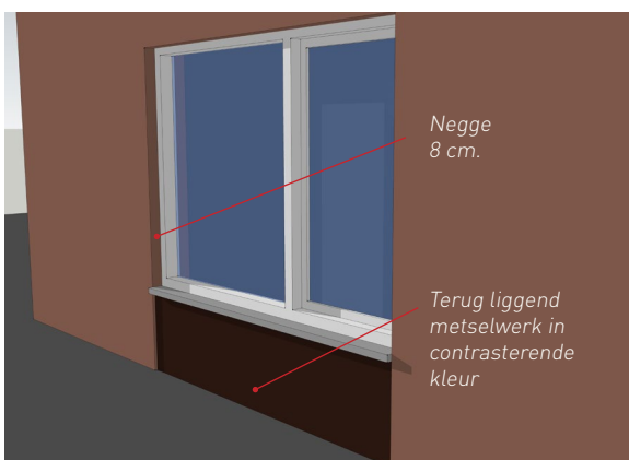
Terugliggend kozijn Metselwerk/paneel in contrasterende kleur Maten en kleuren zijn ter referentie.
